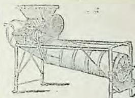
„Триеръ“ за раздѣлине жито и ячменъ отъ ржжъ, къльци и отъ сички нечистотии.
