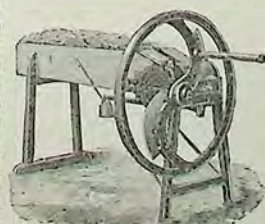
Машина за раздробяване слама.
