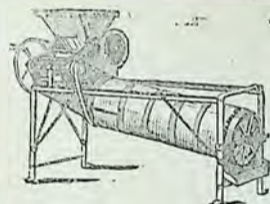
„Триоръ“ за раздѣляние жито и яченикъ отъ ржжъ, кълици и отъ сички нечистоти.
